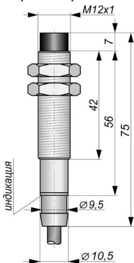
Габаритный чертеж
