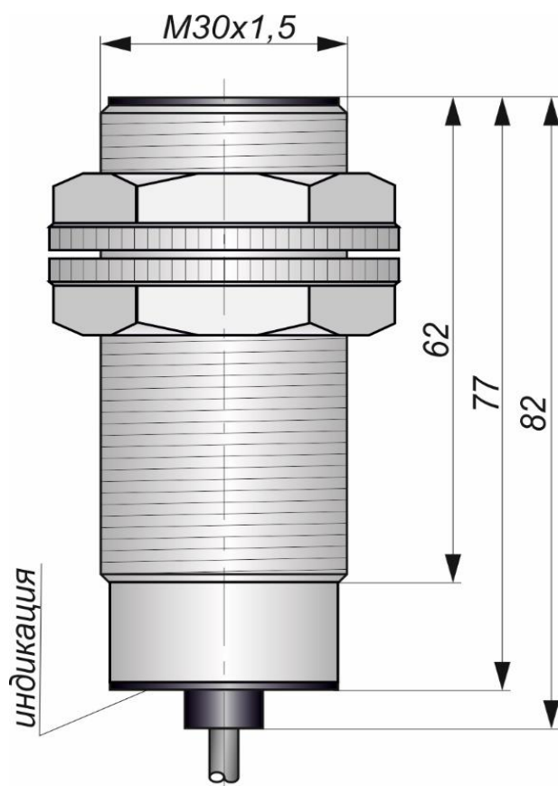
Габаритный чертеж
