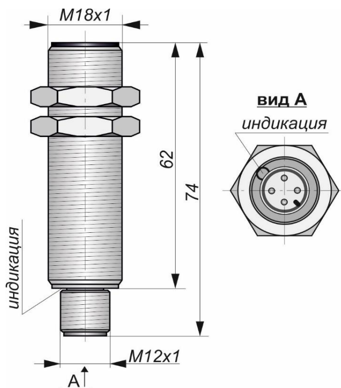
Габаритный чертеж
