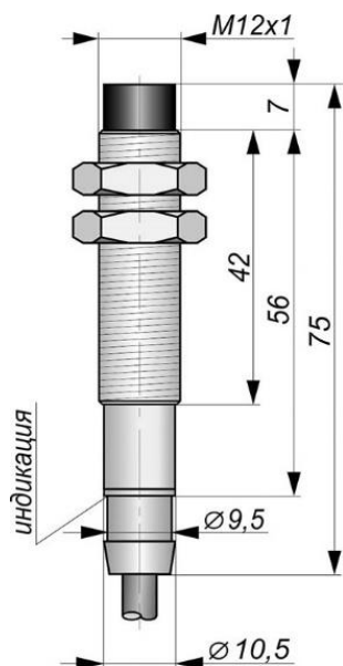
Габаритный чертеж
