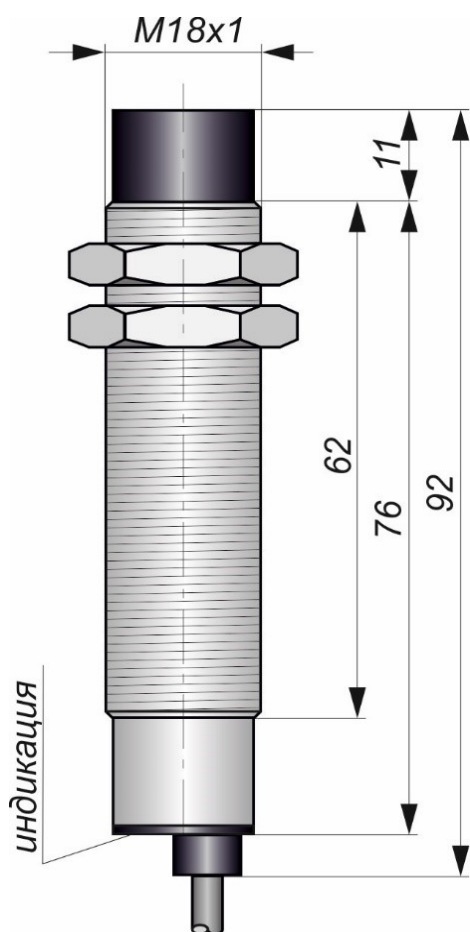
Габаритный чертеж
