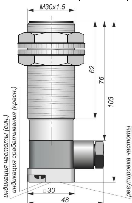
Габаритный чертеж
