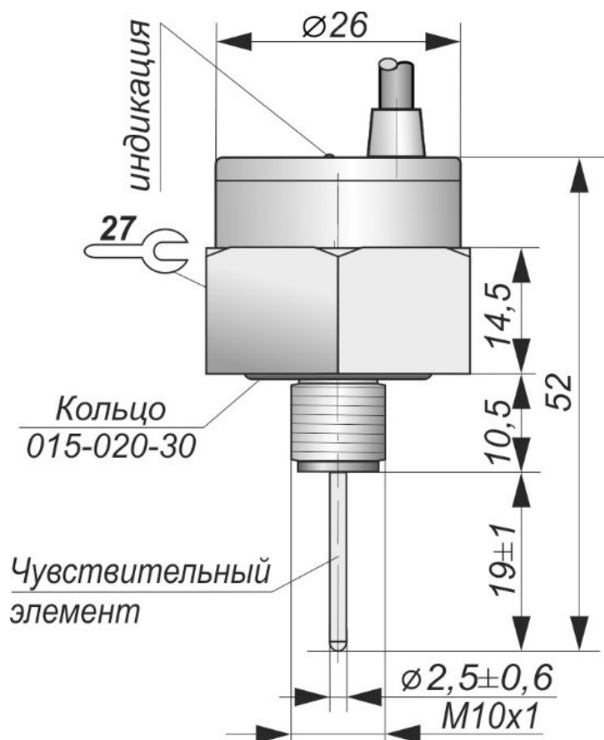
Габаритный чертеж
