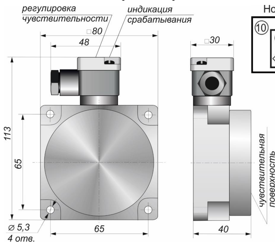
Габаритный чертеж
