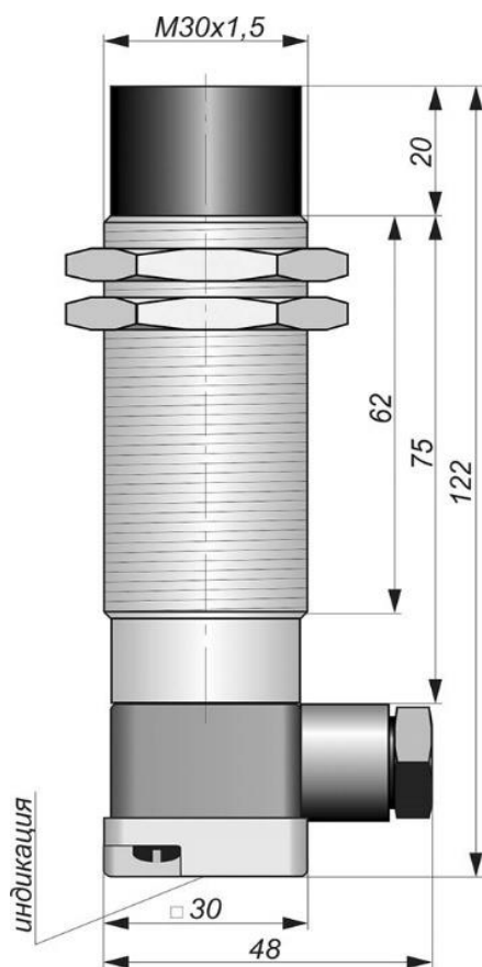
Габаритный чертеж
