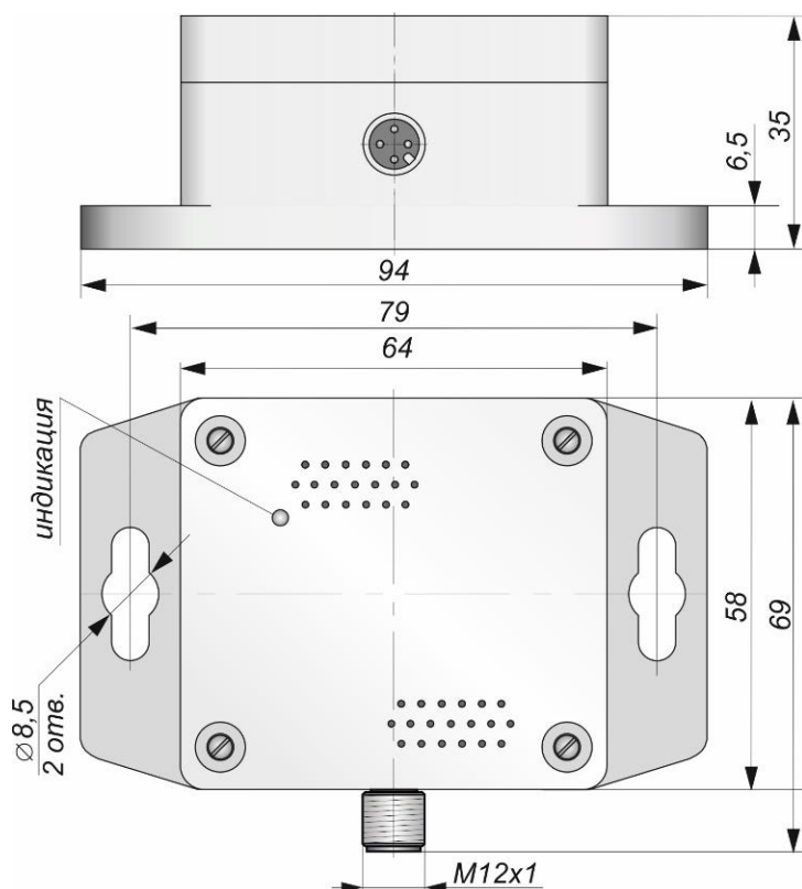
Габаритный чертеж
