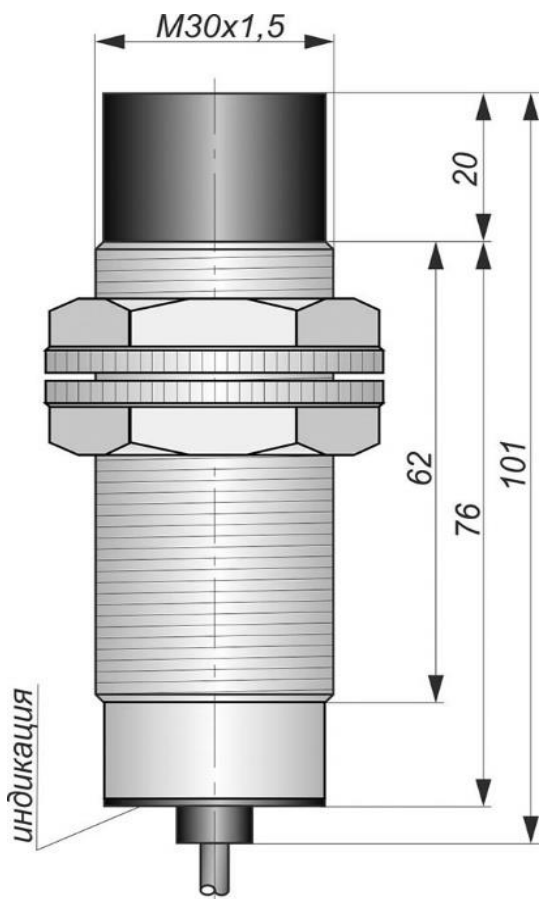
Габаритный чертеж
