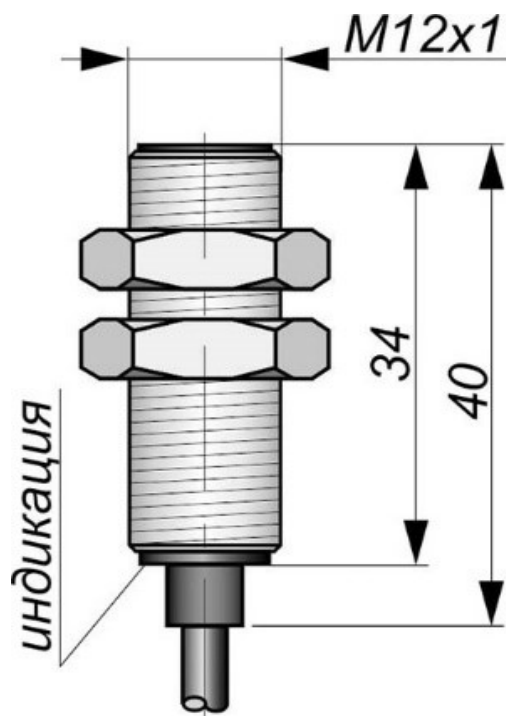
Габаритный чертеж
