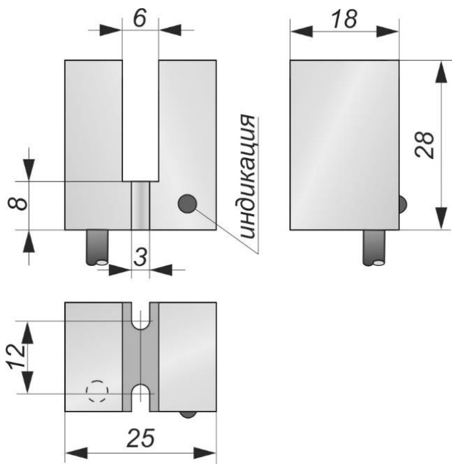
Габаритный чертеж
