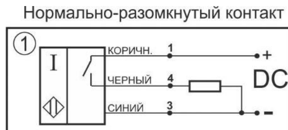
Схема соединения
