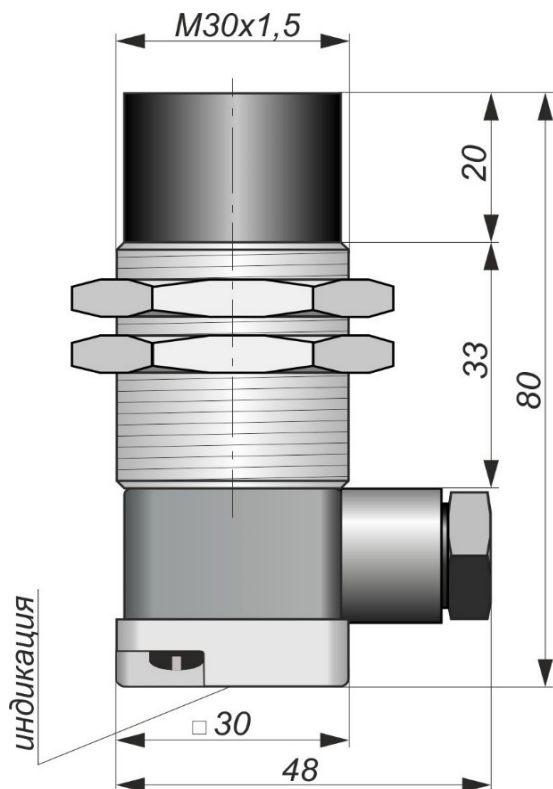
Габаритный чертеж
