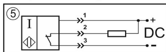
Нормально-замкнутый контакт
