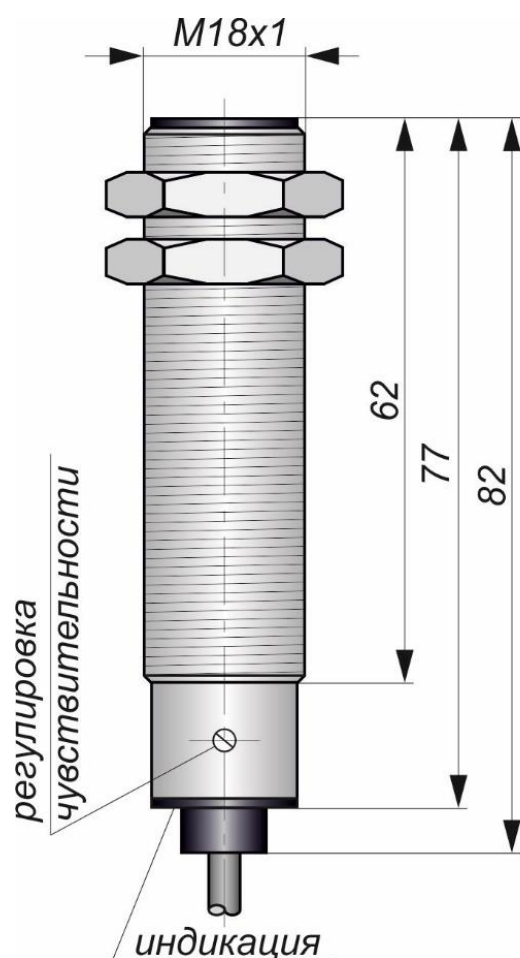
Габаритный чертеж
