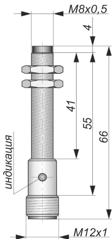
Габаритный чертеж
