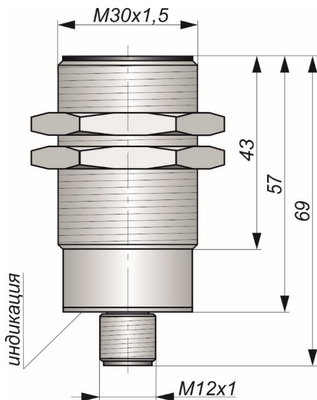
Габаритный чертеж
