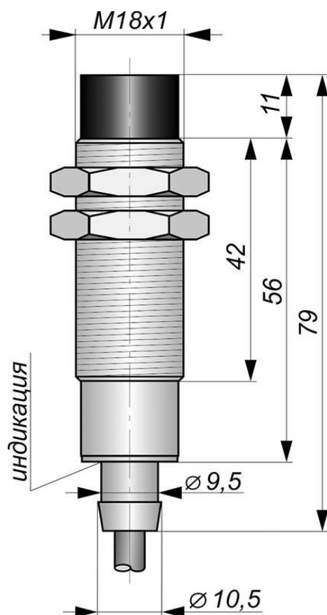
Габаритный чертеж
