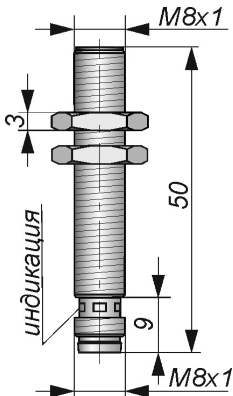
Габаритный чертеж
