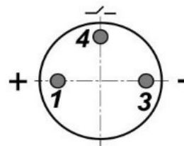
Цоколевка разъема
