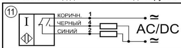
Схема соединения
