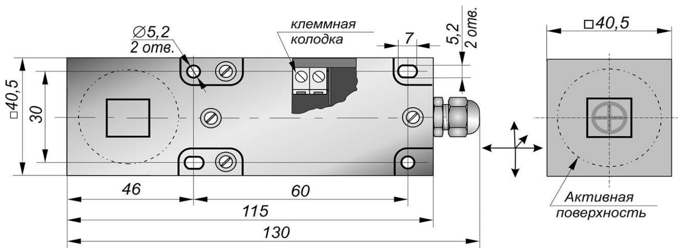
Габаритный чертеж
