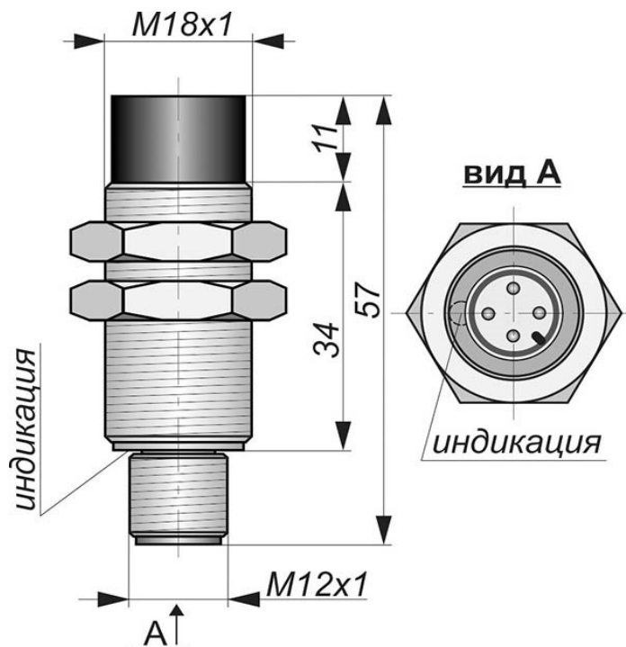
Габаритный чертеж
