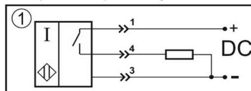
Цоколевка разъема
