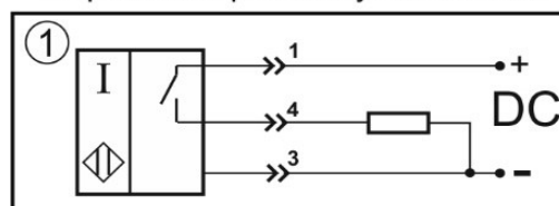
Цоколевка разъема
