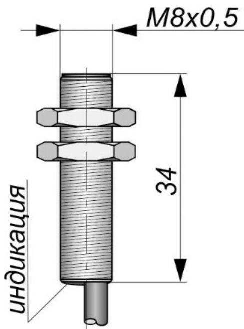
Габаритный чертеж
