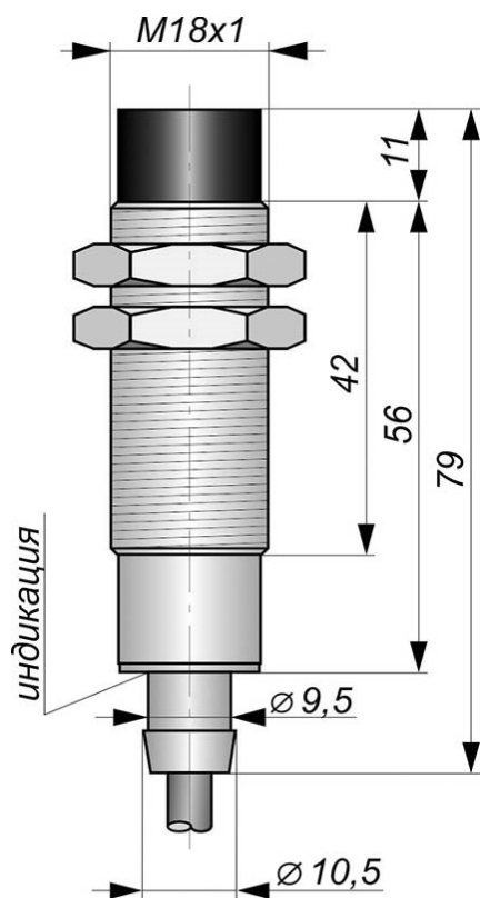
Габаритный чертеж
