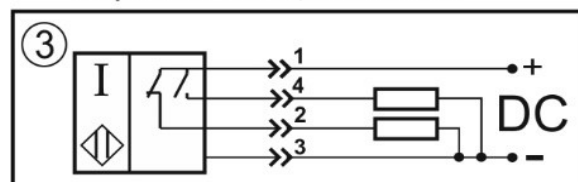
Схема соединения Переключающий контакт
