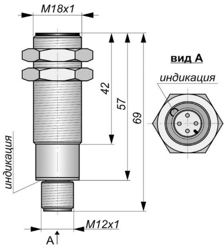
Габаритный чертеж
