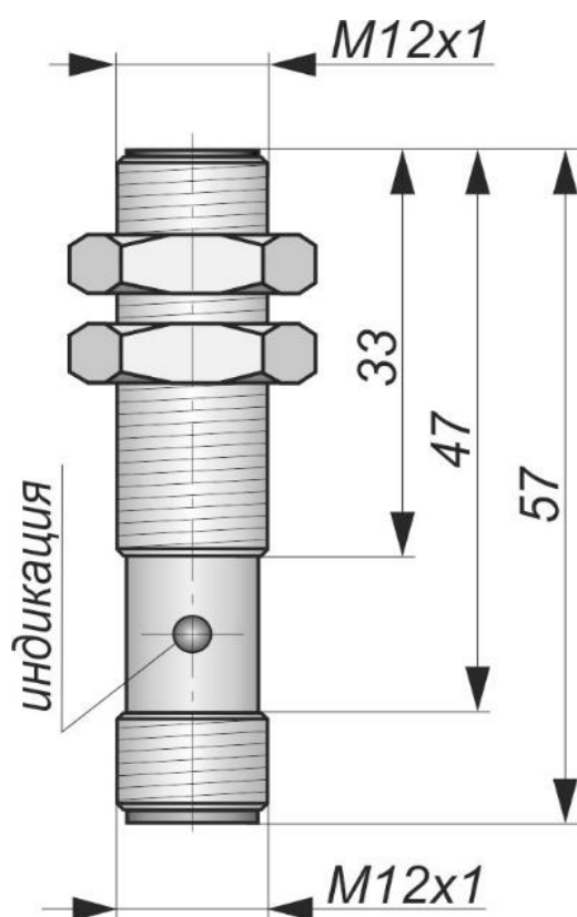
Габаритный чертеж
