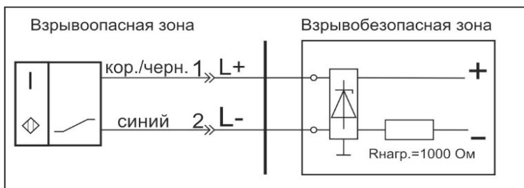
Схема соединения
