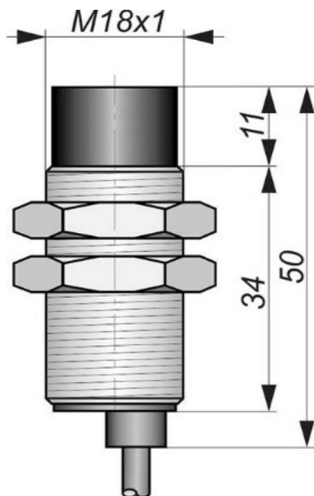
Габаритный чертеж
