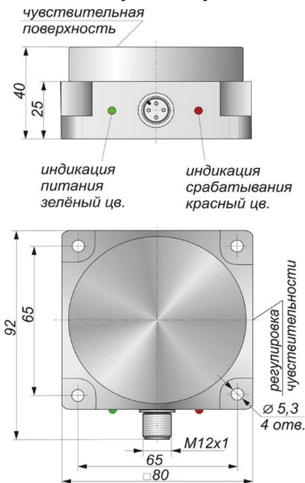
Габаритный чертеж
