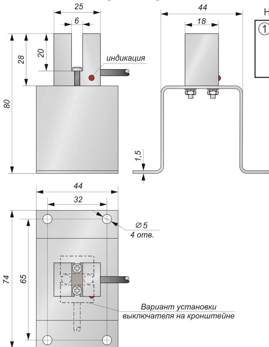
Габаритный чертеж
