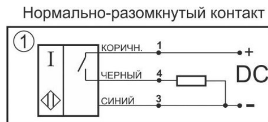
Схема соединения
