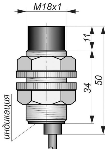
Габаритный чертеж
