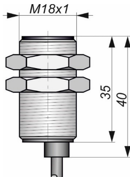
Габаритный чертеж
