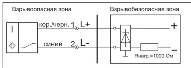
Схема соединения
