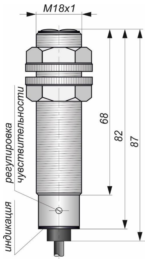
Габаритный чертеж
