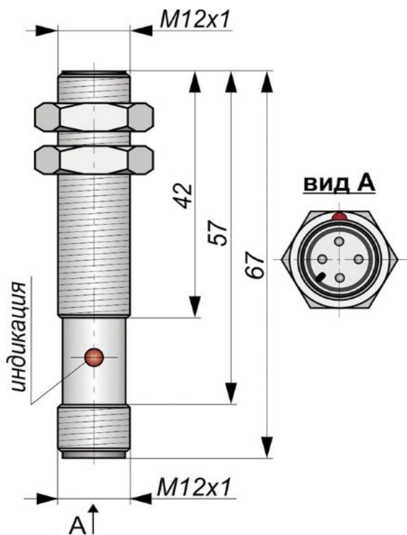
Габаритный чертеж
