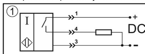
Цоколевка разъема
