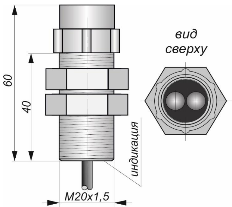
Габаритный чертеж
