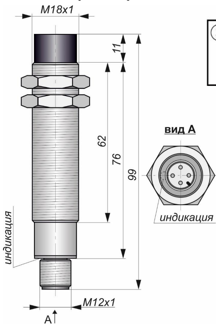
Габаритный чертеж
