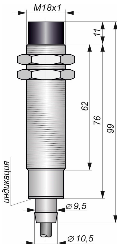
Габаритный чертеж
