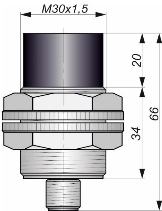
Габаритный чертеж
