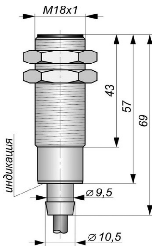
Габаритный чертеж
