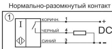
Схема соединения
