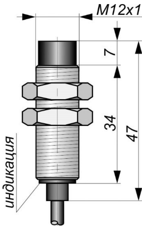
Габаритный чертеж
