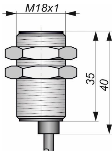
Габаритный чертеж
