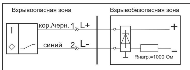
Схема соединения
