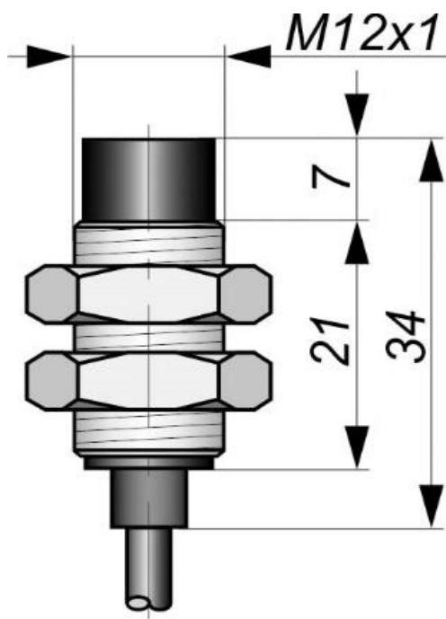
Габаритный чертеж
