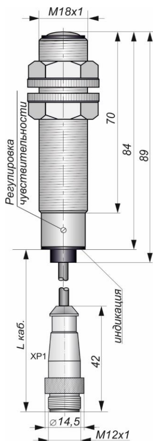
Габаритный чертеж
