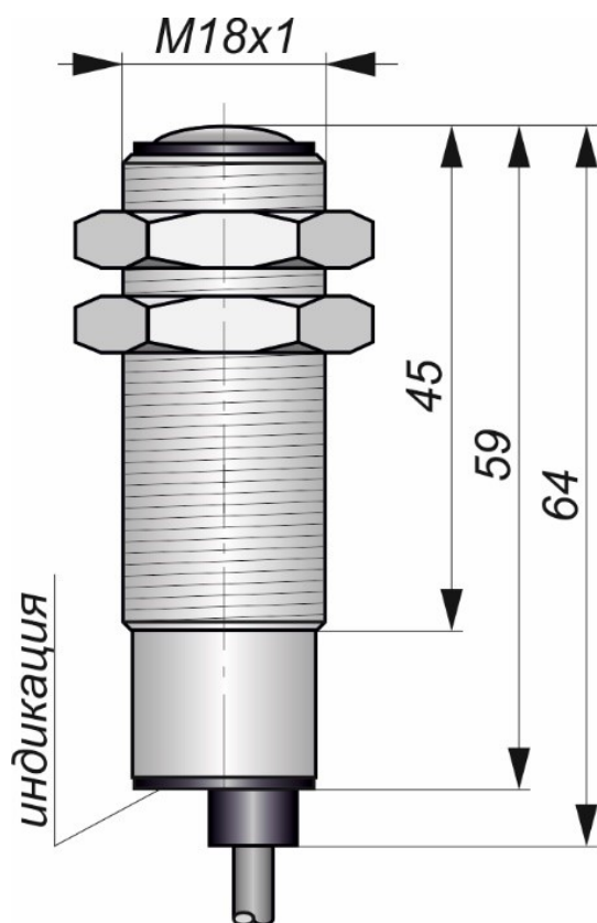
Габаритный чертеж
