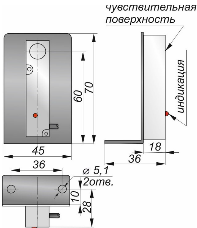
Габаритный чертеж
