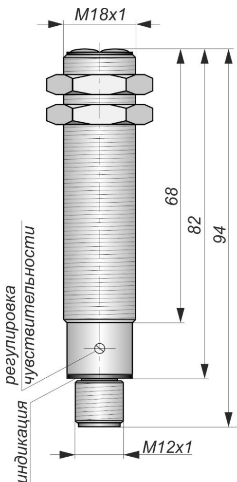
Габаритный чертеж
